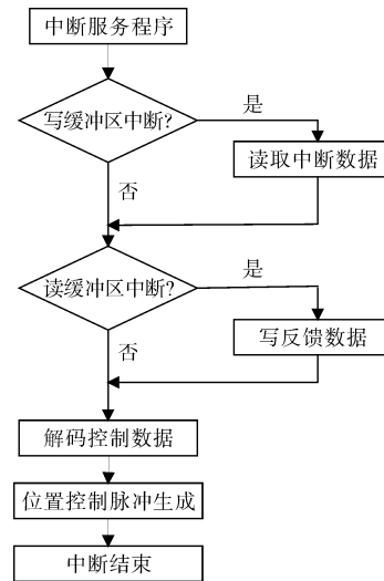
图 6 程序中断流程图
