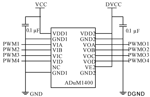
图 3 电机隔离电路
