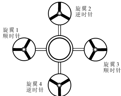
图 1 小型四旋翼飞行器结构俯视图
